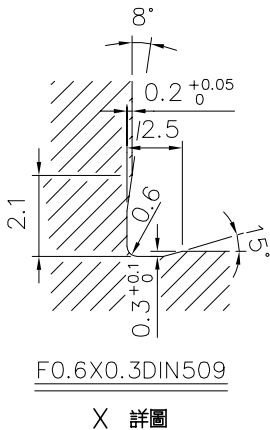
X 詳圖
