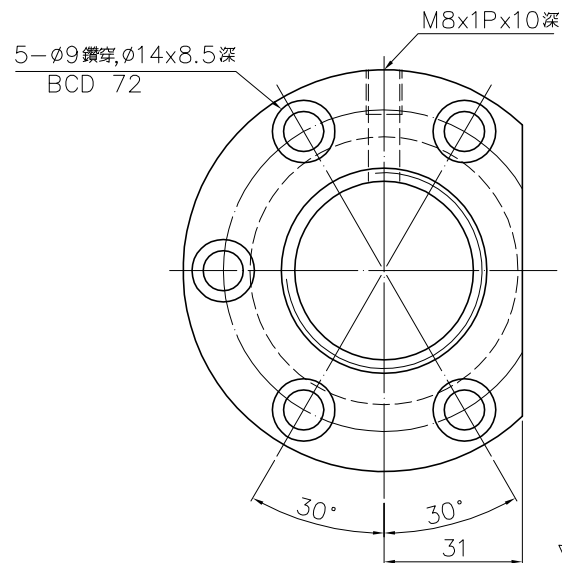
D-D 視圖
